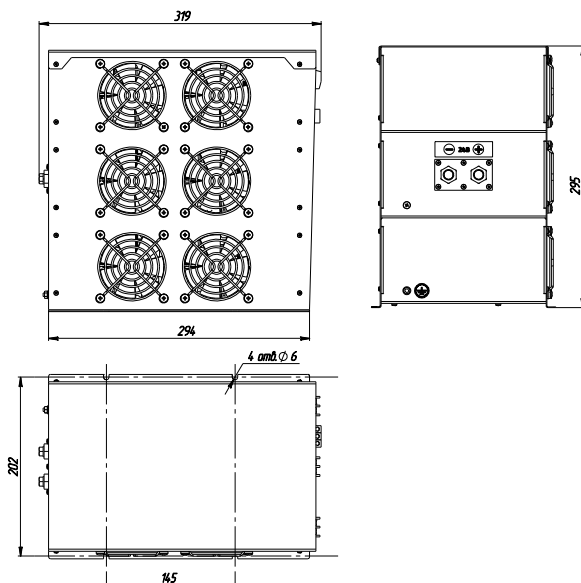
Рис.1.3 ИС1-24-6000У2 (вид изделия)
